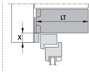
Abb. B – Anputzblech, Laibungs-/Sturzkanal (4)
