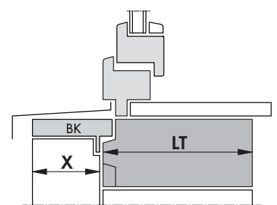
Abb. C – Brüstungskanal (BK) (4)
